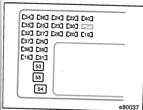
Panoul de instrumente (vehicule cu volanul pe partea dreapta)
