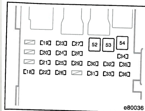
Panoul de instrumente (vehicule cu volanul pe partea stânga)
