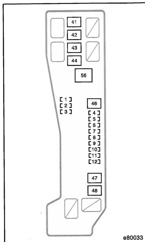
Compartimentul motorului (motor pe benzină)
