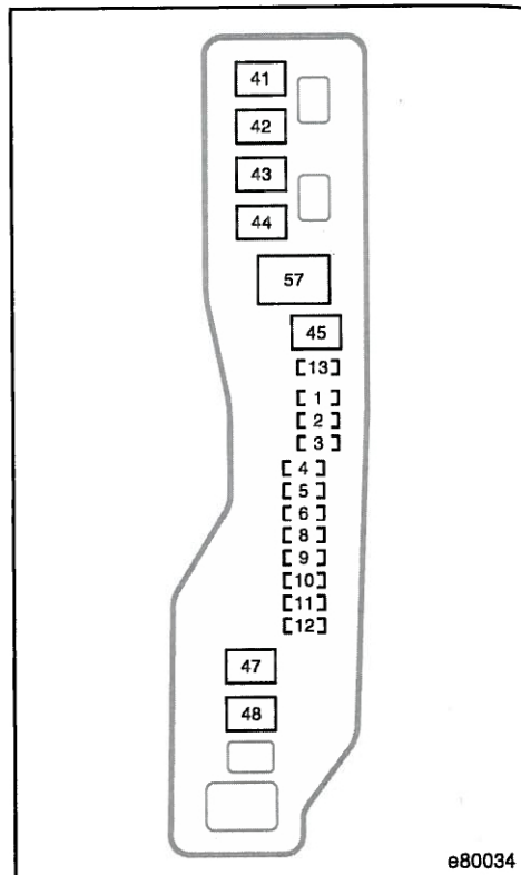
Compartimentul motorului (motor diesel)
